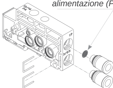
Filtro std. su alimentazione (P)
