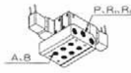
Uscite inferiori
