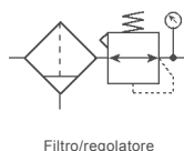
Filtro/regolatore
